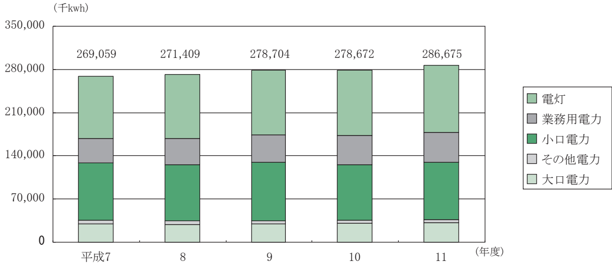
図3-15 電力需要の推移
