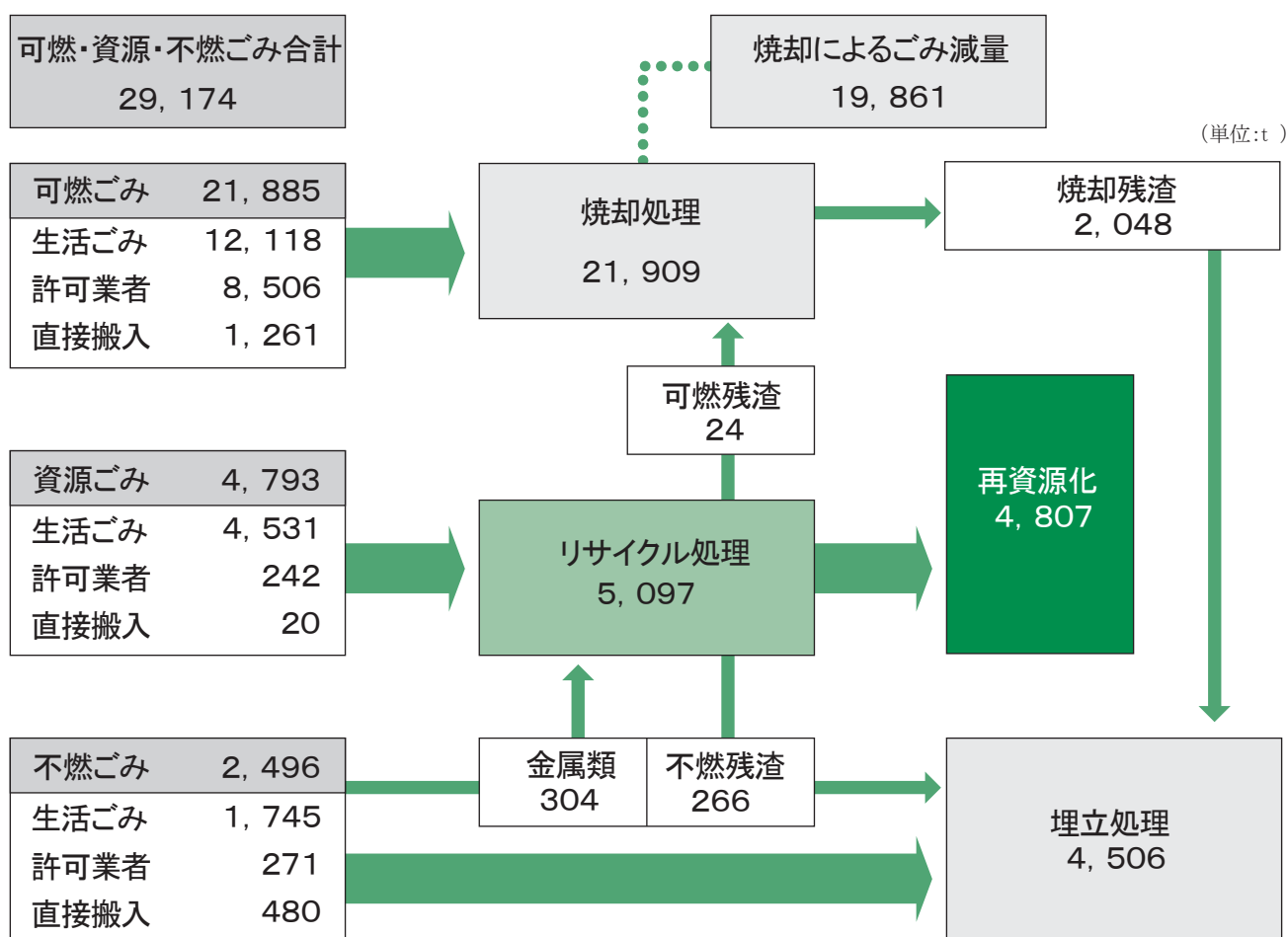
図3-14 ごみ処理フローシート(平成13年度)
