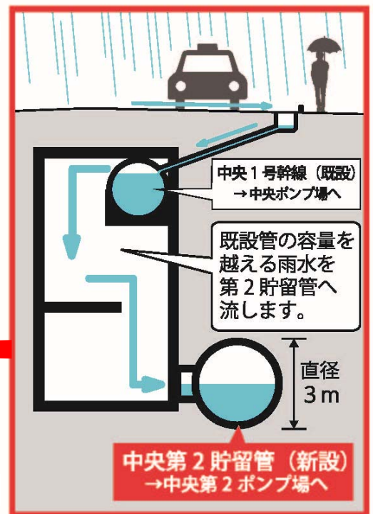
中央第 2 貯留管の断面図
