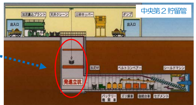
▲雨水貯留管となるトンネルのイメージ
