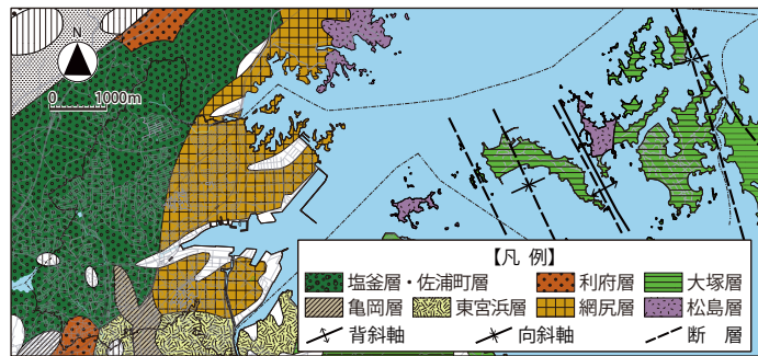
図 1-3 塩竈市周辺の地質図
