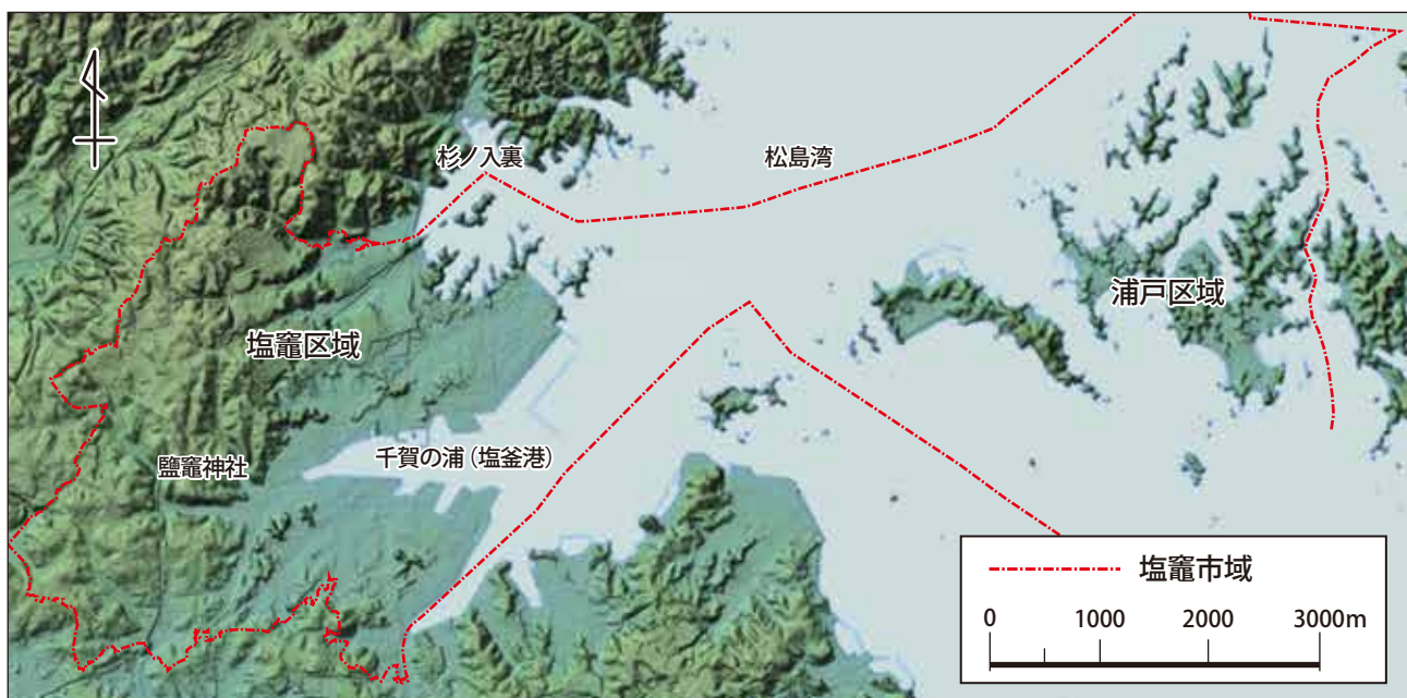
図 1-4 塩竈市の起伏図
