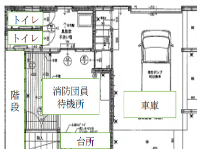
1F 平面図
