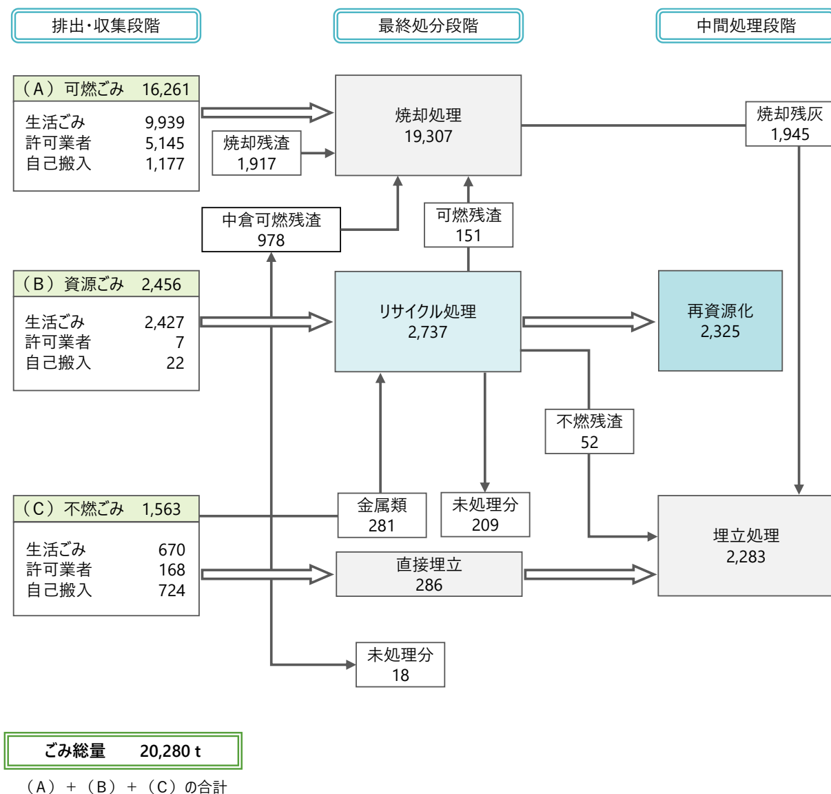
【ごみ処理フローシート（令和4年度実績）】
