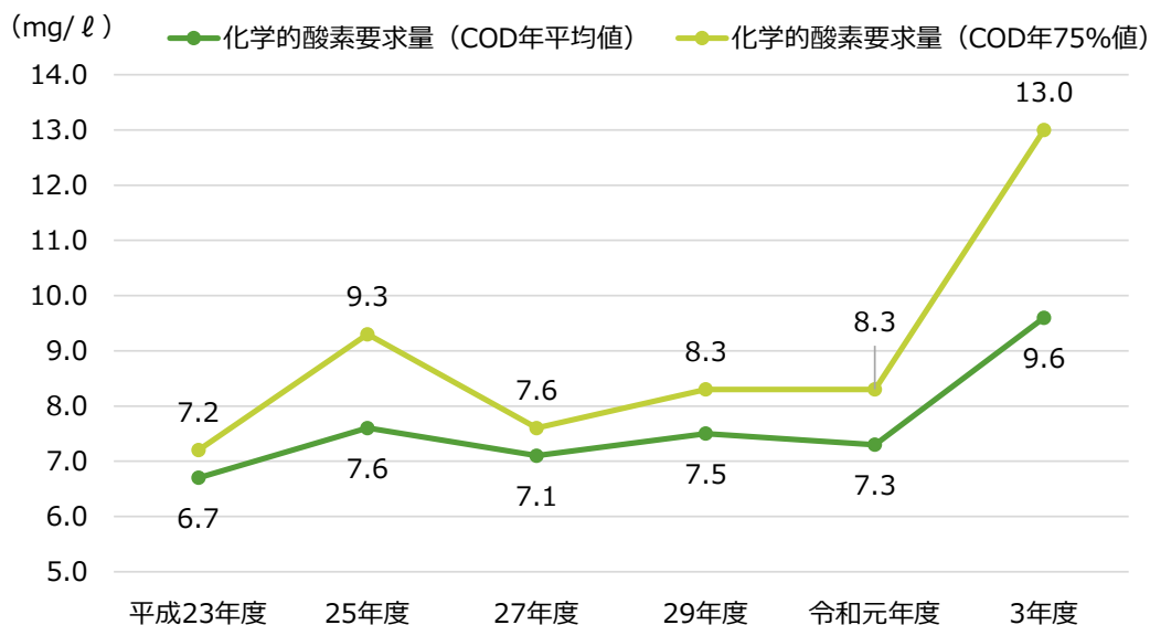
【加瀬沼のCOD（化学的酸素要求量）年平均値の推移】
