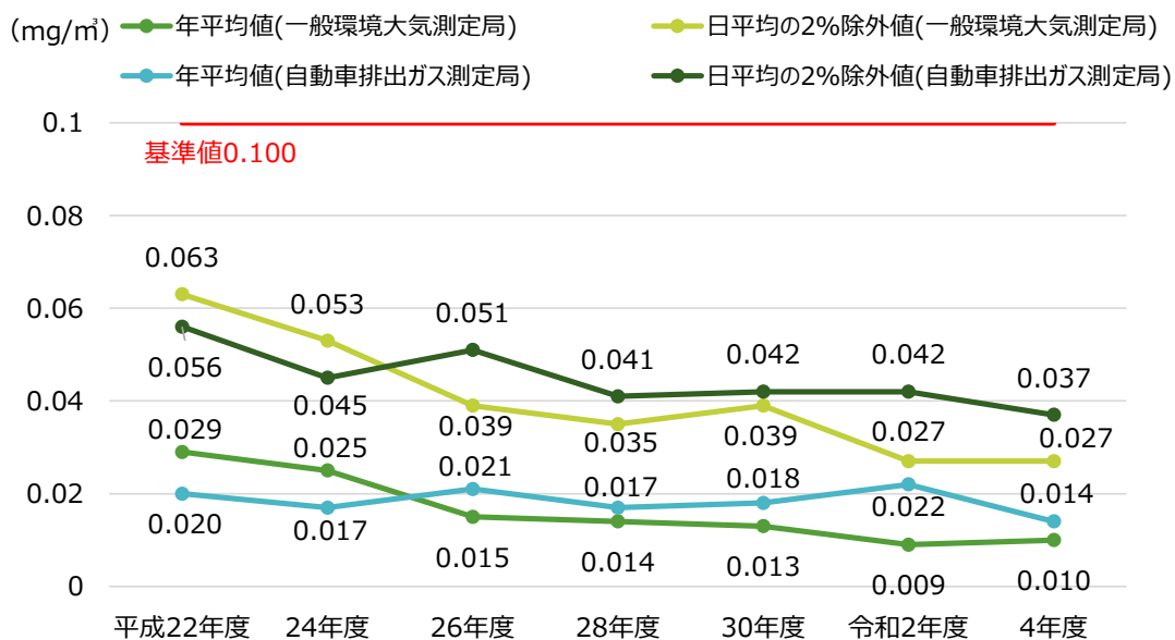
【浮遊粒子状物質濃度の推移】
