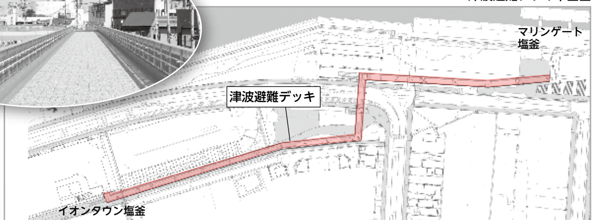
▼津波避難デッキ平面図
