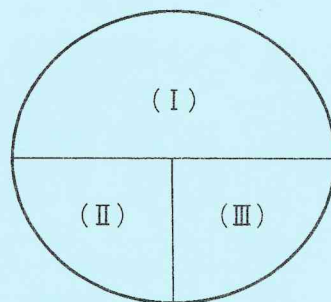
図2 速さの公式
