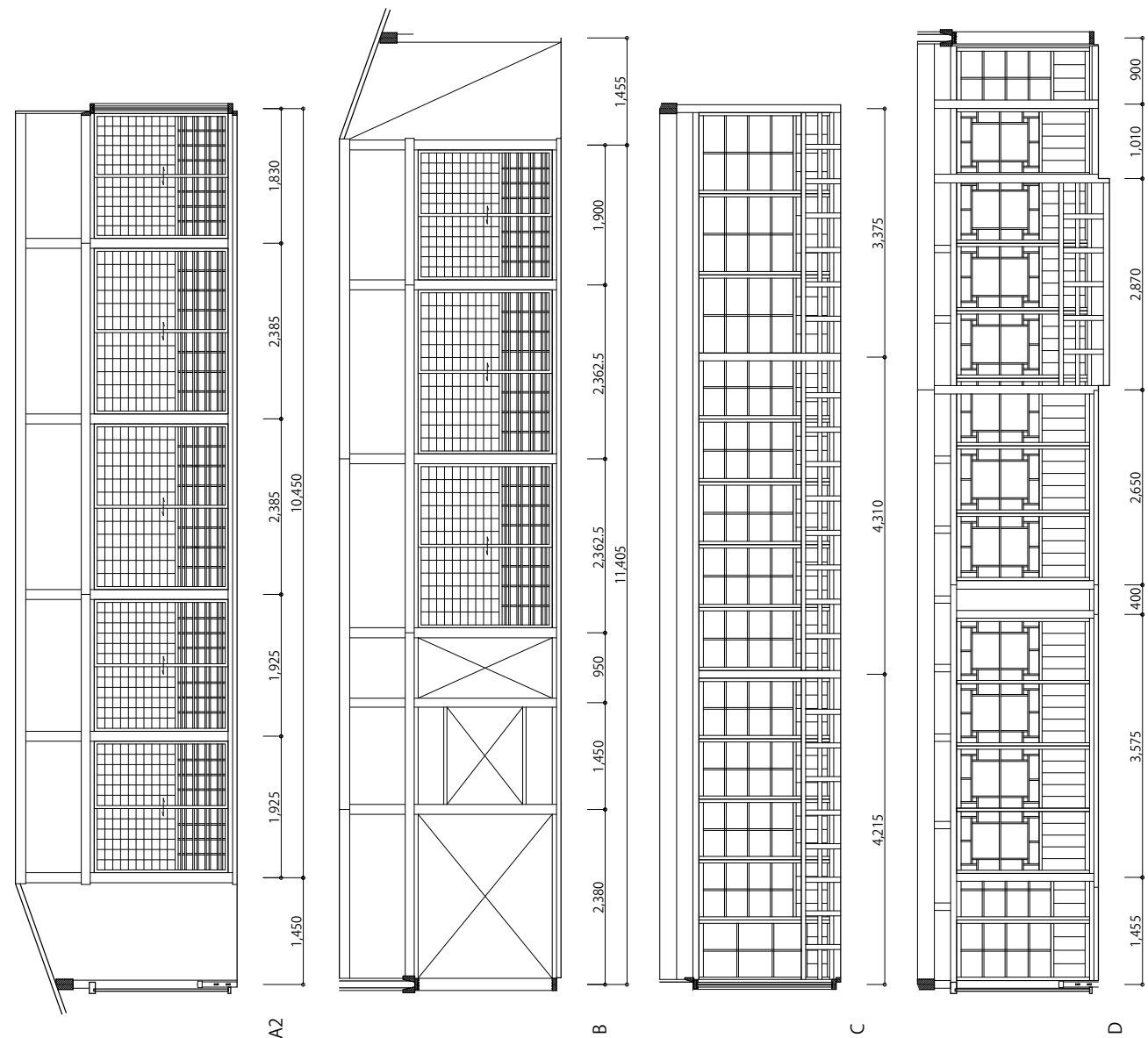
第18図 展開図8(縁側)
