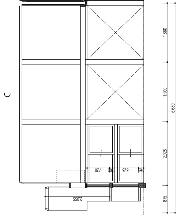
第11図 展開図1 (広間棟広間(18畳間、御成之間))
